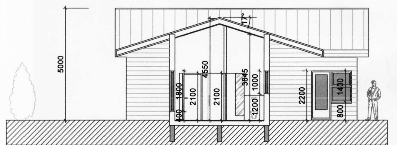
SNEIÐING Y-Y 1:100
