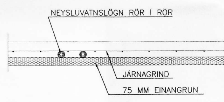
SNID Í NEYSLUVATNSLÖGN RÖR Í RÖR 1:20
