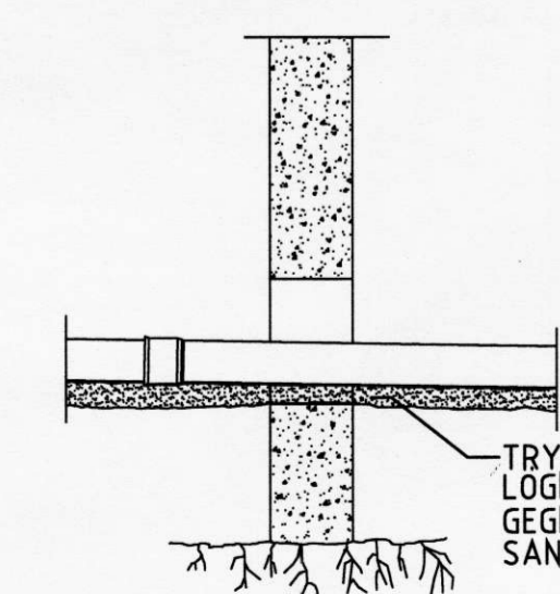
DÆMIGERT SNIÐ Í FRÁGANG LAGNA Í GEGNUM SÖKKULVEGGI, M 1:20
