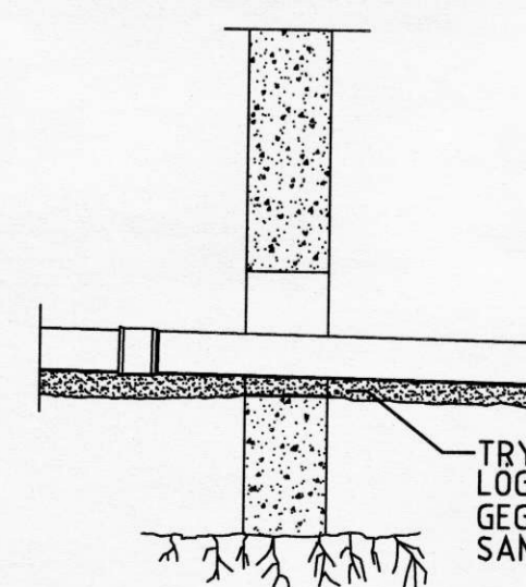
DÆMIGERT SNID Í FRÁGANG LAGNA Í GEGNUM SÖKKULVEGGI, M 1:20
