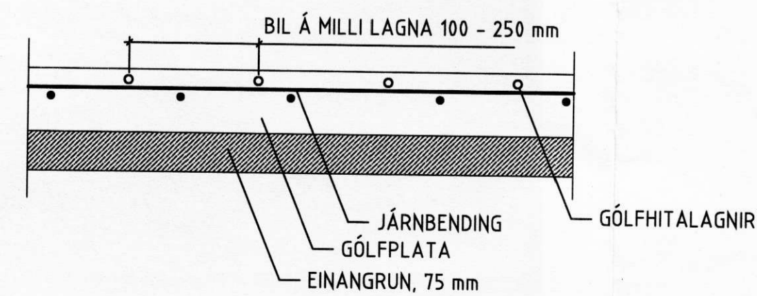
SNÍÐ Í GÓLFHITALÖGN 1. HÆÐ, MKV. 1:10
