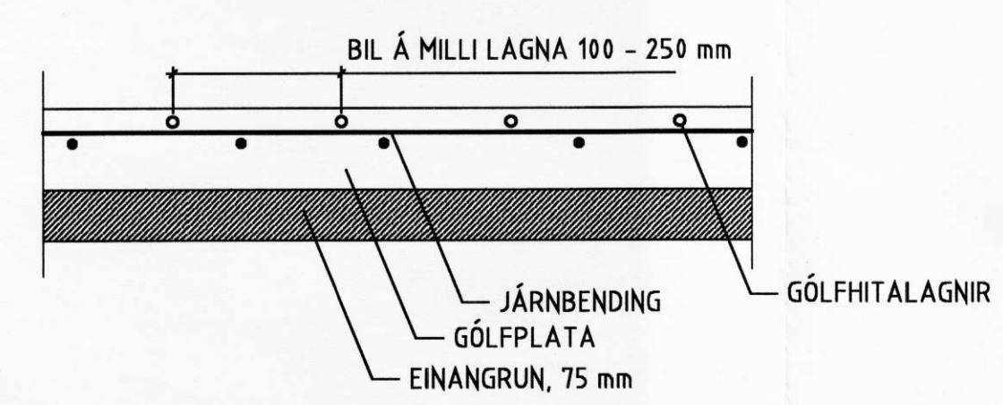
SNID Í GÓLFHITALÖGN 1. HÆÐ, MKV. 1:10
