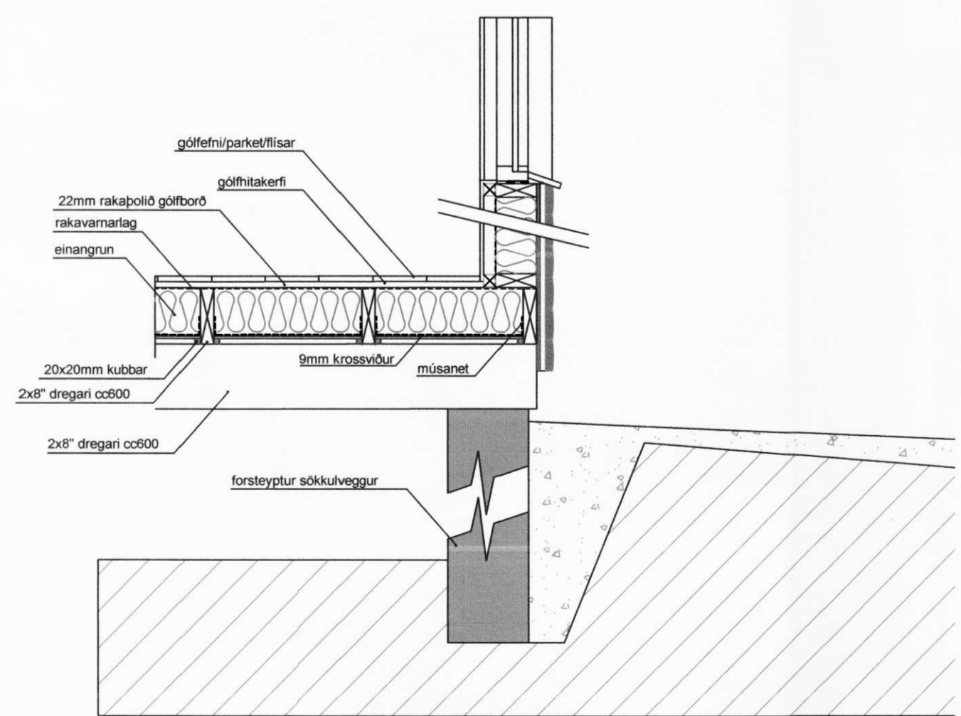
SNEIÐING Z-Z 1:50
