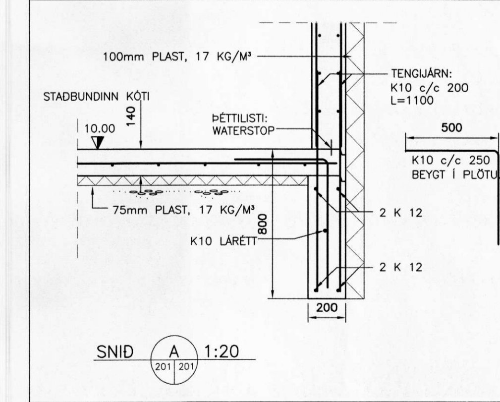
GRUNDUN Mkv. 1:50
