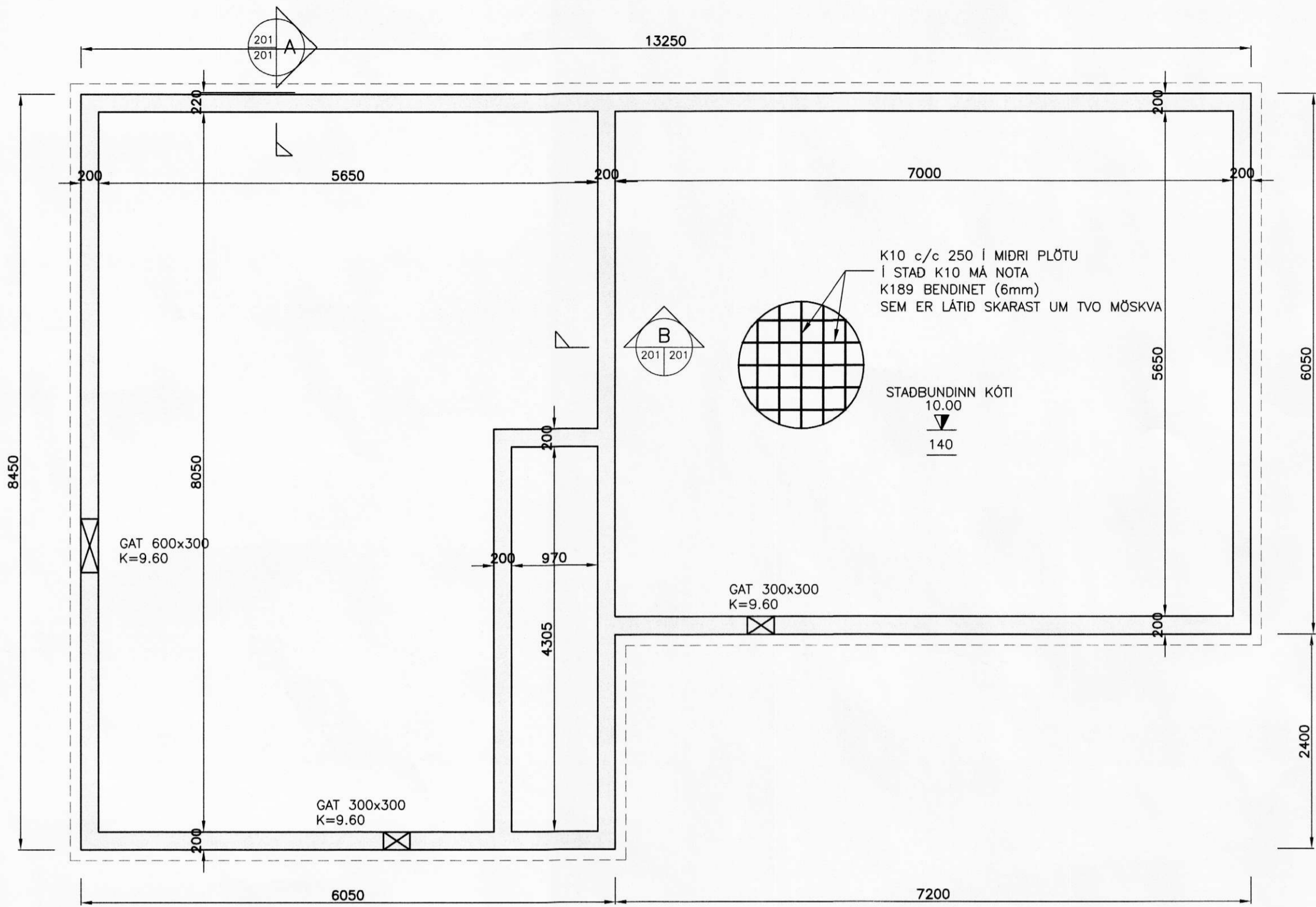
GRUNNMYND SÖKKULS MKV. 1:50
