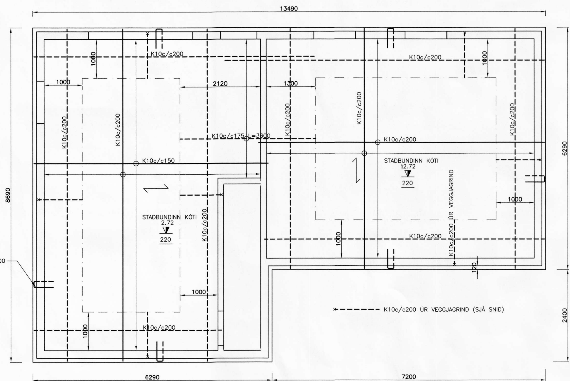
GRUNNMYND PLÖTU MKV. 1:50
