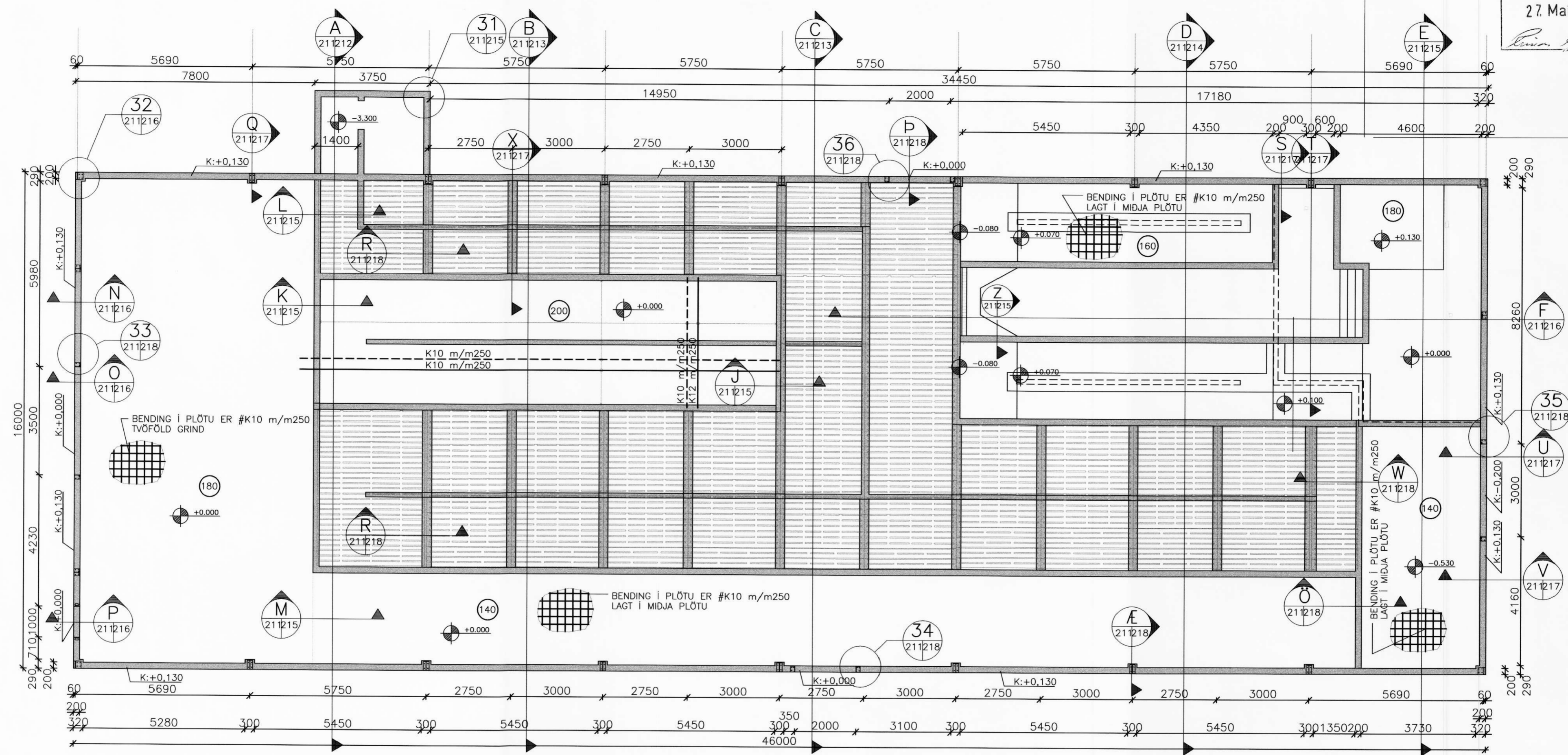
GRUNNMYND 1:100
