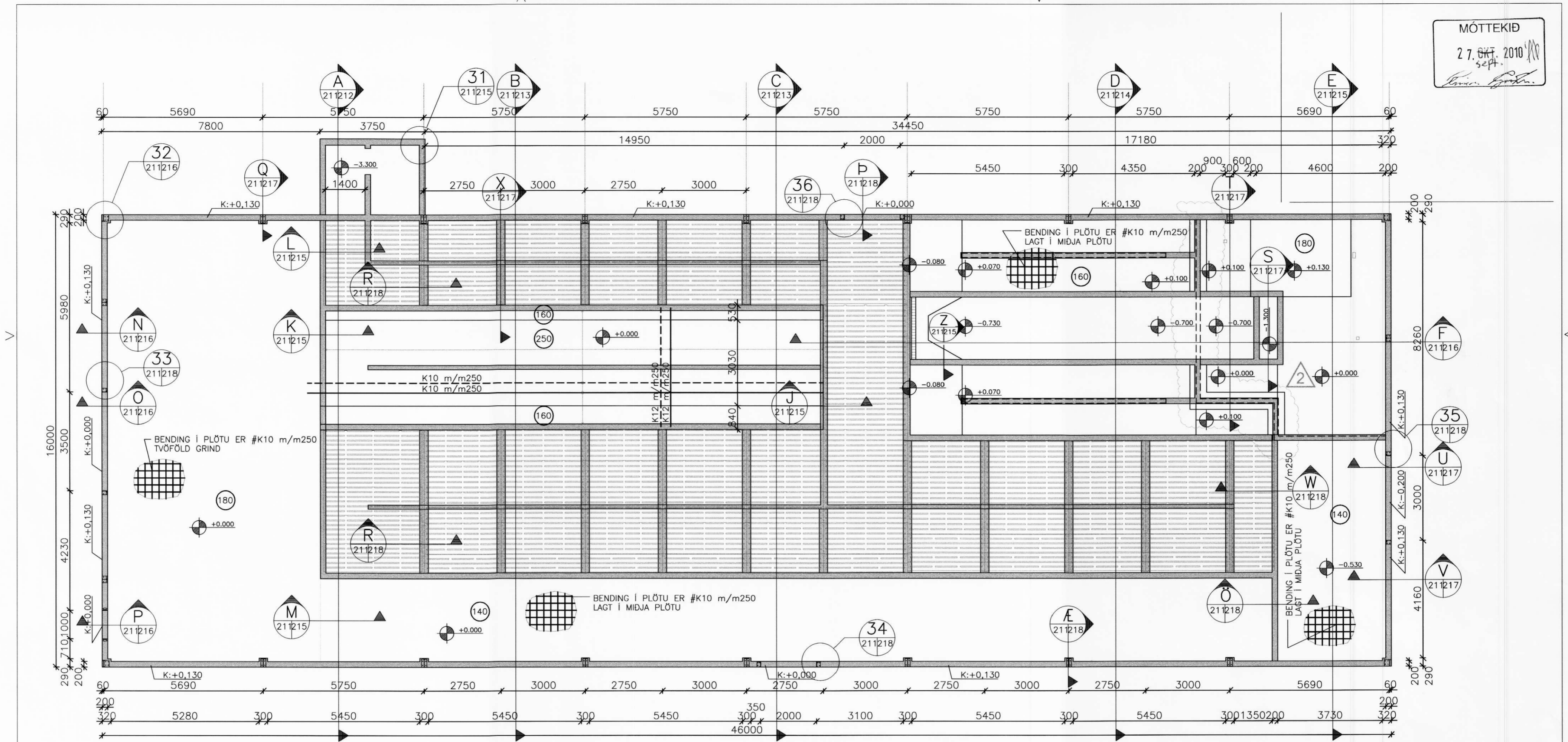
GRUNNMYND 1:100
