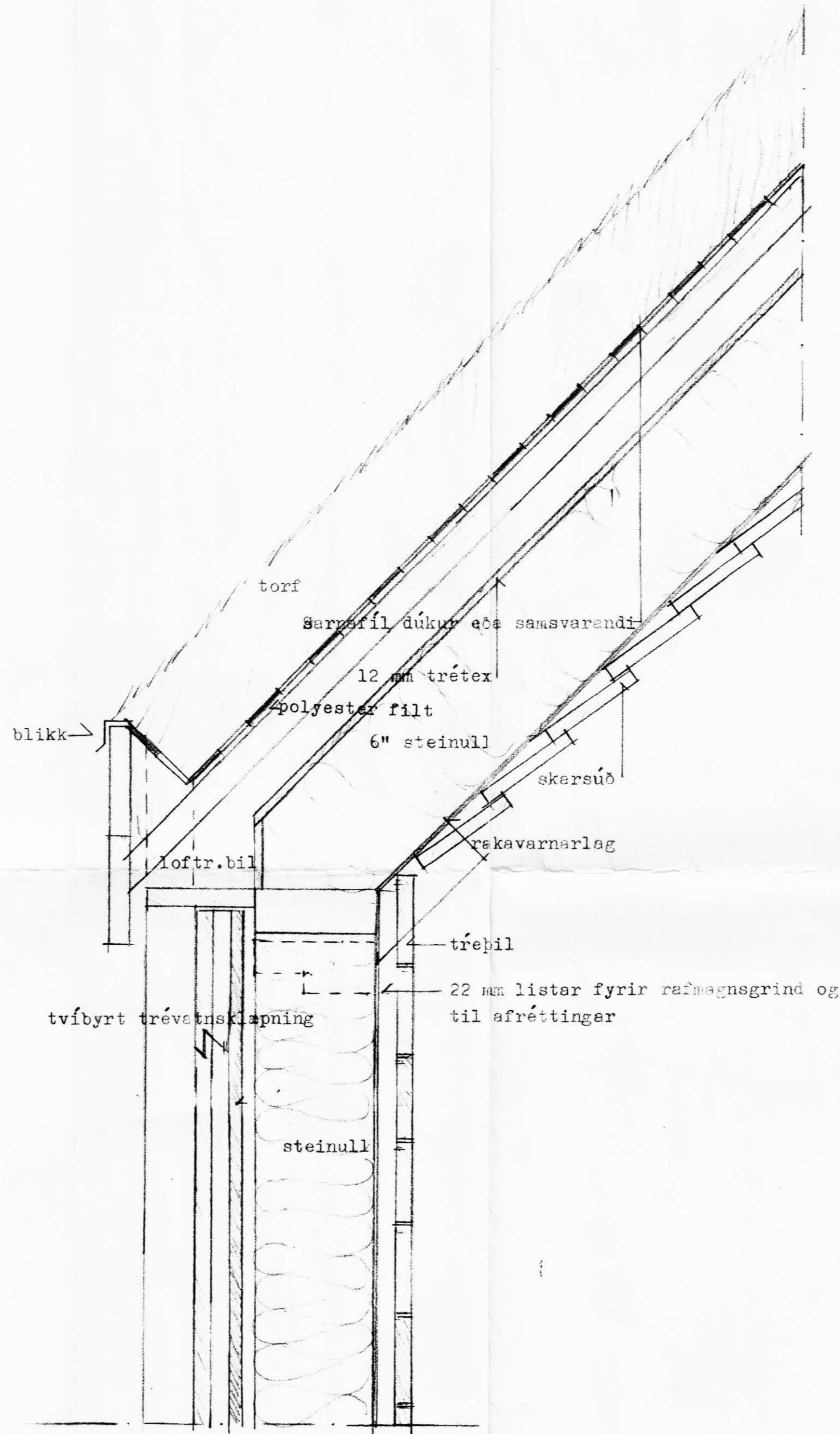
Þakskegg í tengibyggingu á einangruðum vegg og glervegg ( rofin lína gluggapósts)
