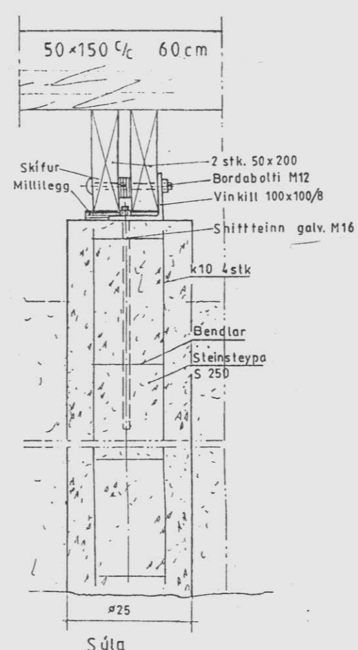
C-C
