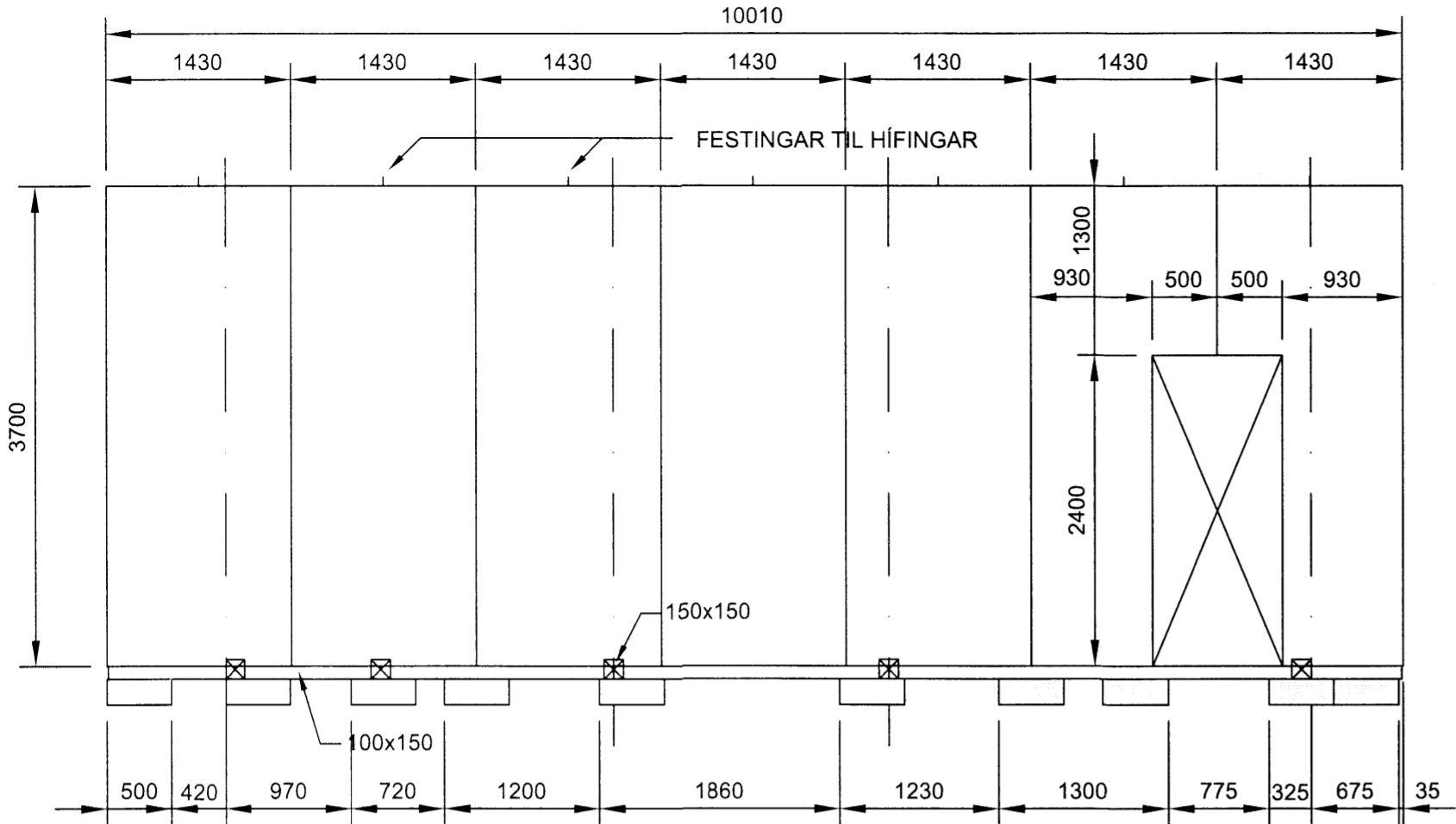
BRUNAVARNAVEGGUR Í MÁTLÍNU O - ÁSÝND 1:50
