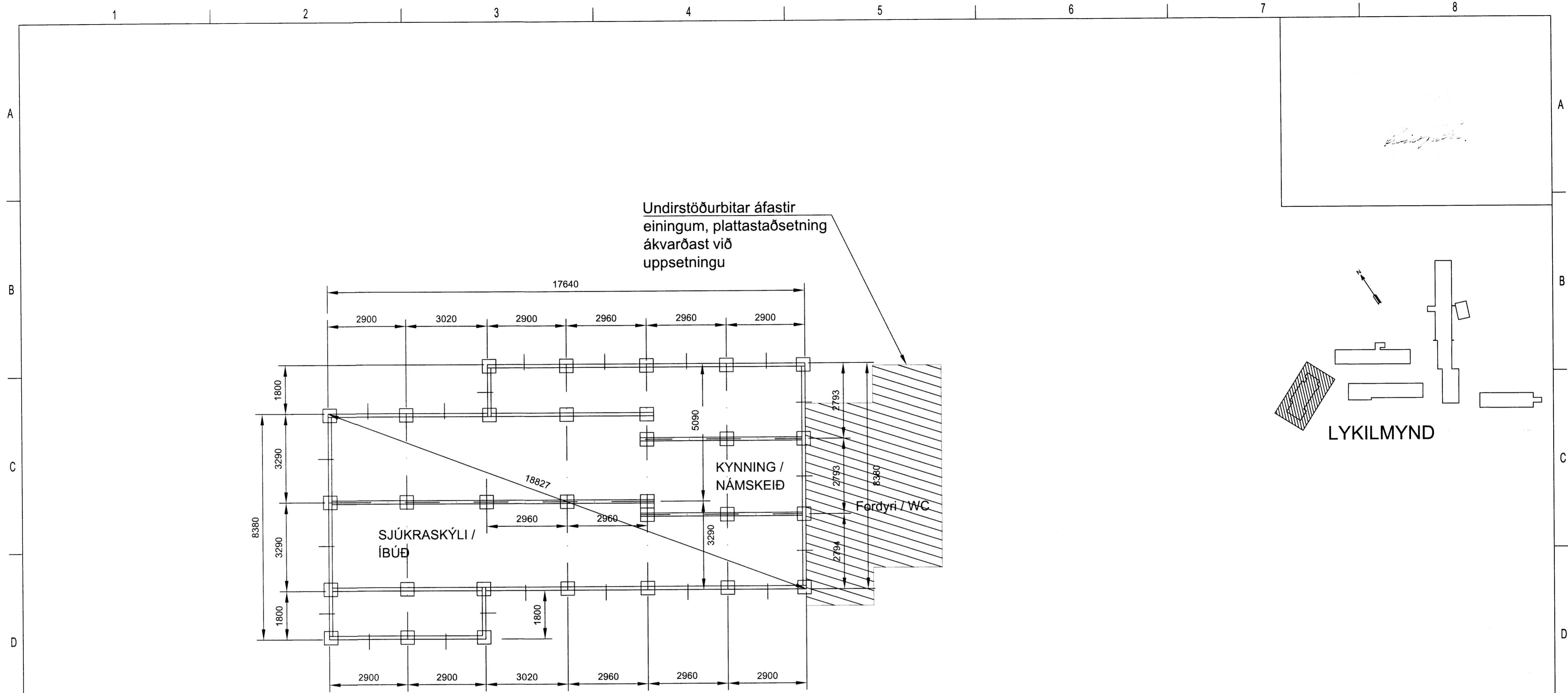
SJÚKRASKÝLI OG KYNNING, GRUNNMYND MKV. 1
