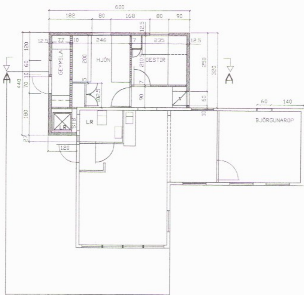
GRUNNMYND
