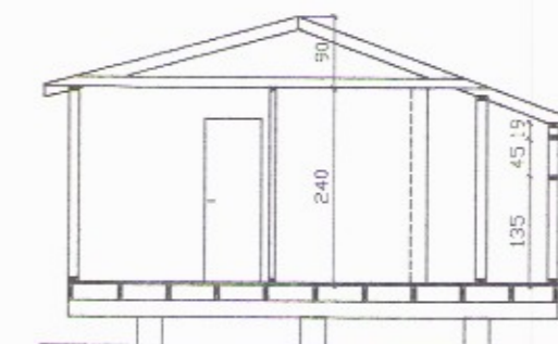
SNEIÐING A-A
