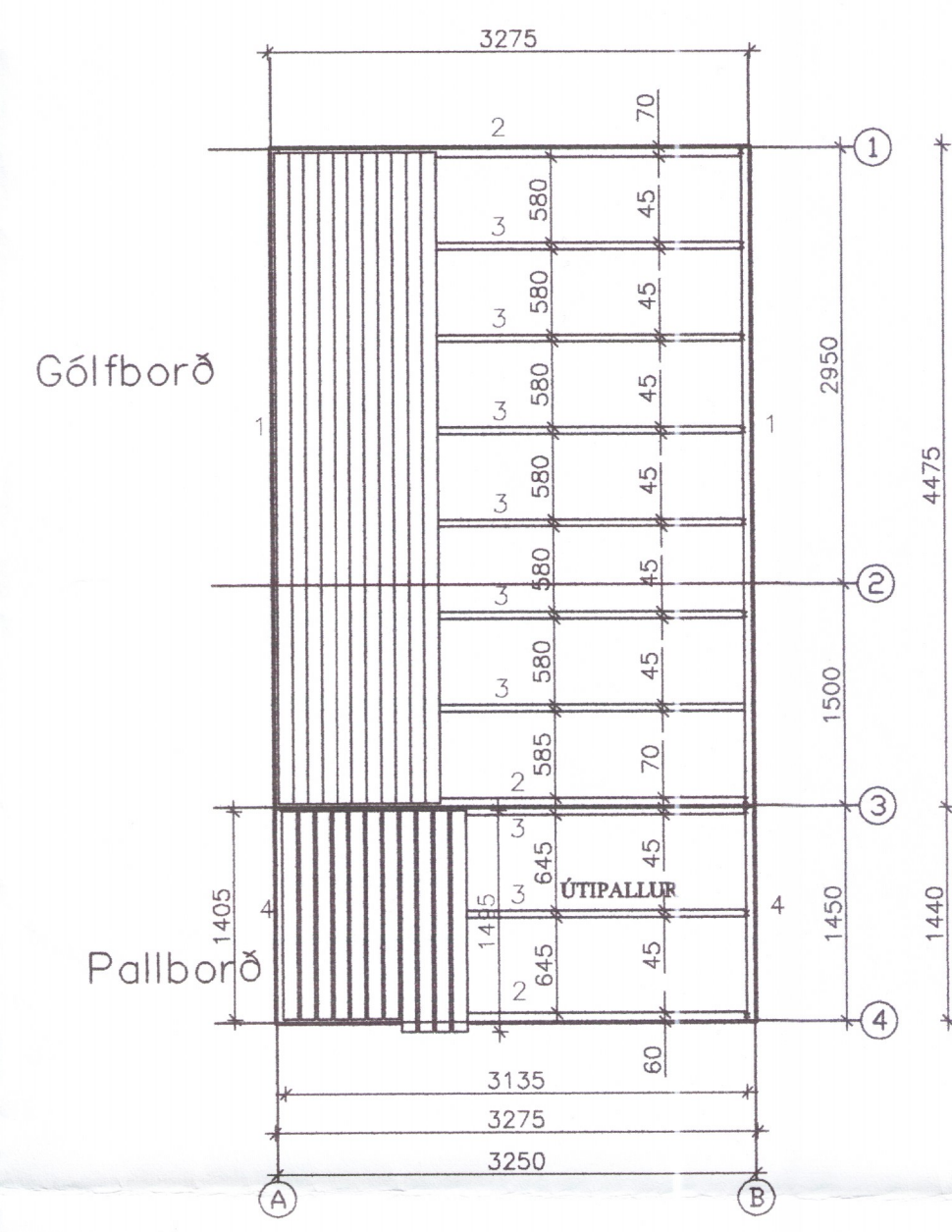
Grunnmynd gólfborð
