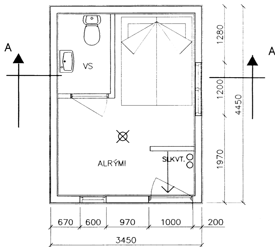
GRUNNMYND 1:50
