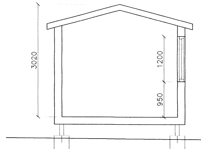
SNID A-A 1:50
