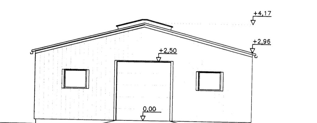
VESTUR HLID
