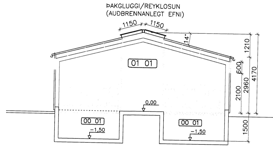
SNEIDING
