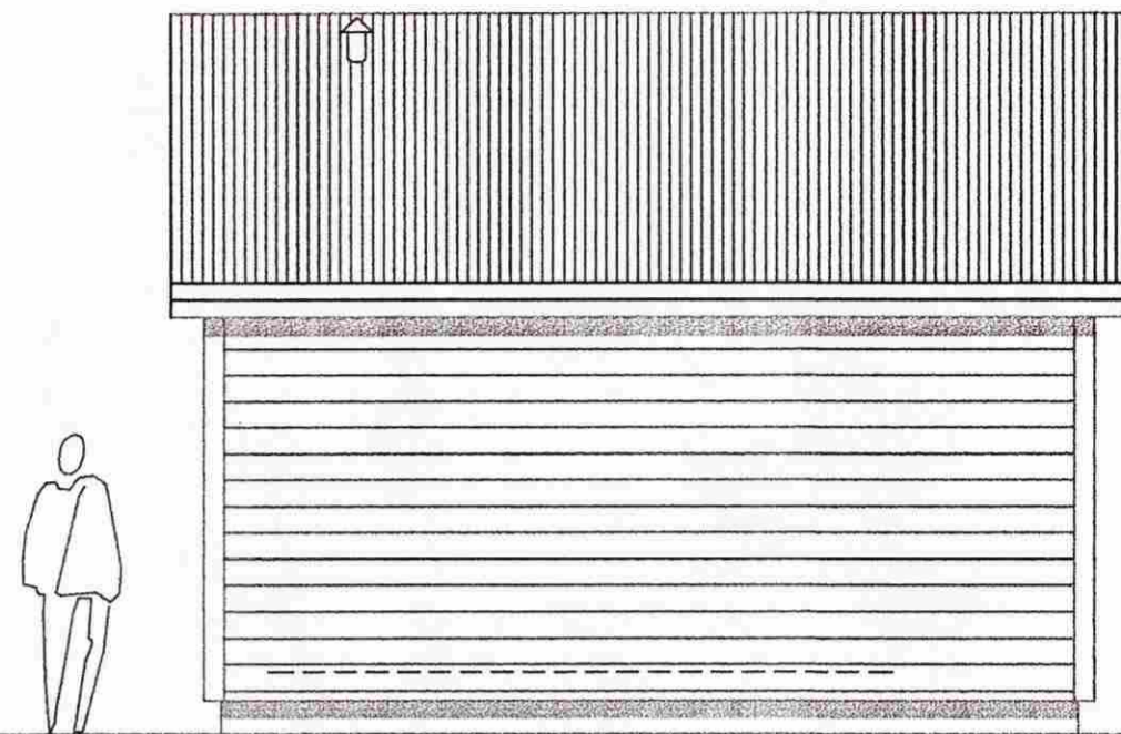
SUDURHLID 1:50
