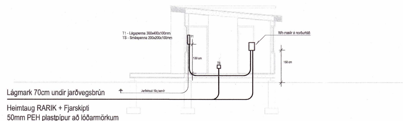
SNID um inntak M 1:100
