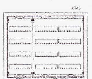
LÁGSPENNU- OG SMÁSPENNUHÖLF STRIEBEL & JOHN AT43
