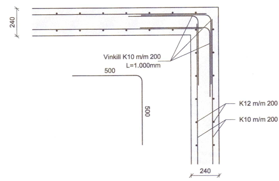
I Deili 120-01 M 1:20
